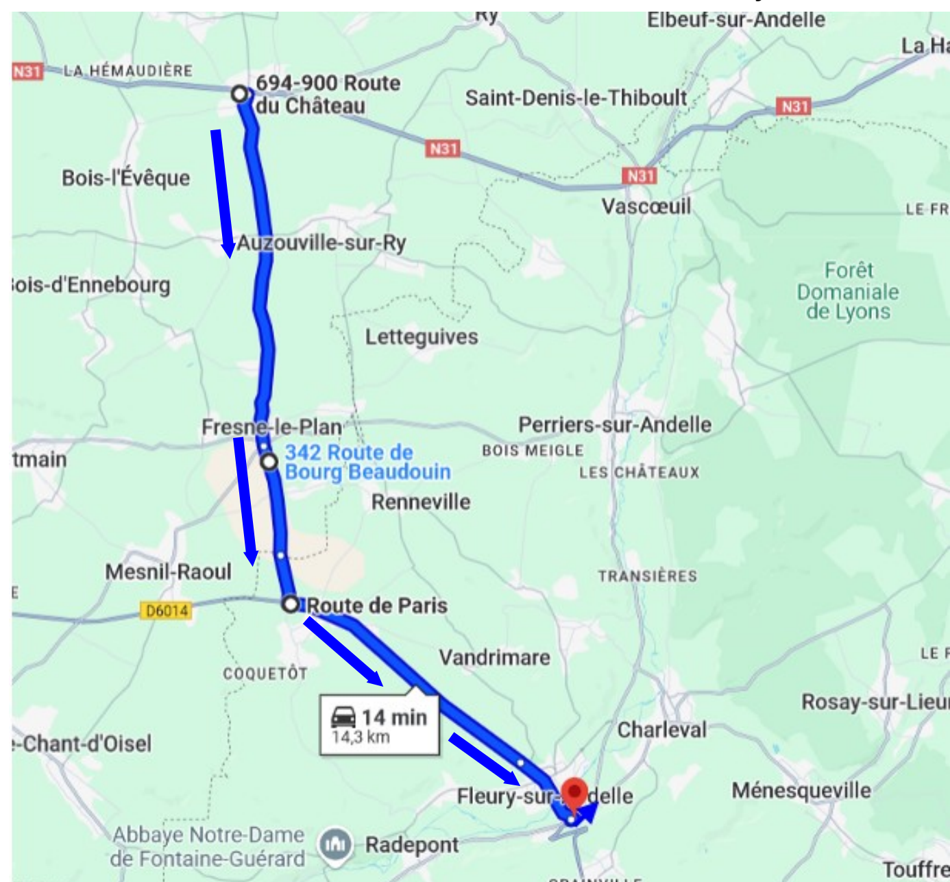
Plan de déviation sens Rouen vers Gournay
